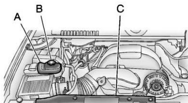
Двигатель 5300 V8 (для двигателя 6000 V8 – аналогично)
