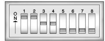
Пример панели с восемью трехпозиционными переключателями
